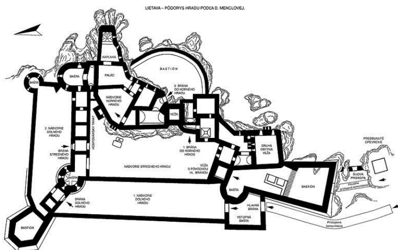
Pódorys hradu Lietava.
