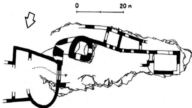
Pôdorys Starého hradu.
