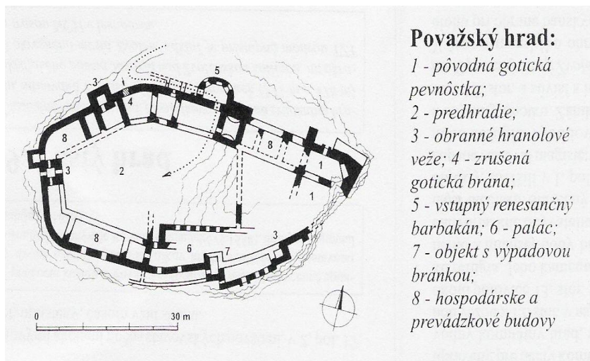
Pôdorys Považského hradu.
