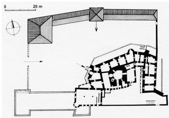
Pôdorys
